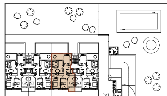
PLANTA SEGUNDA
